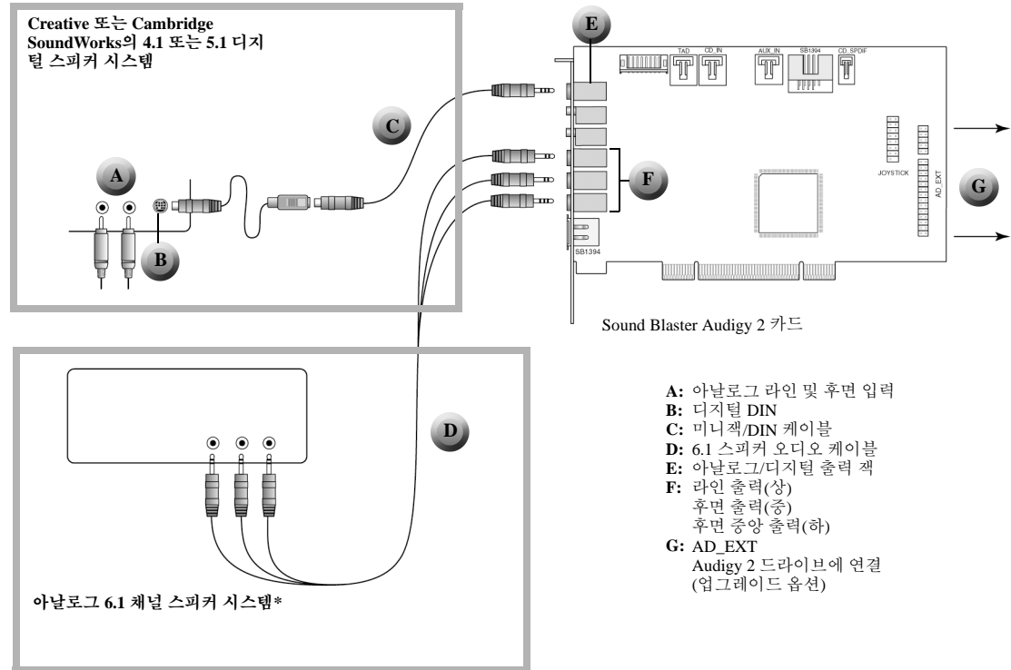
그림 1-8: 스피커 시스템에 Sound Blaster Audigy 2 카드 연결하기
