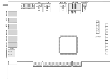
Sound Blaster Audigy 2 카드
