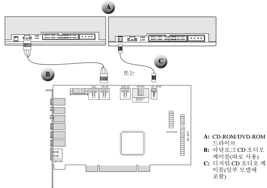
그림 1-6: CD-ROM/DVD-ROM 드라이브에 아날로그/디지털 오디오 케이블 연결하기
