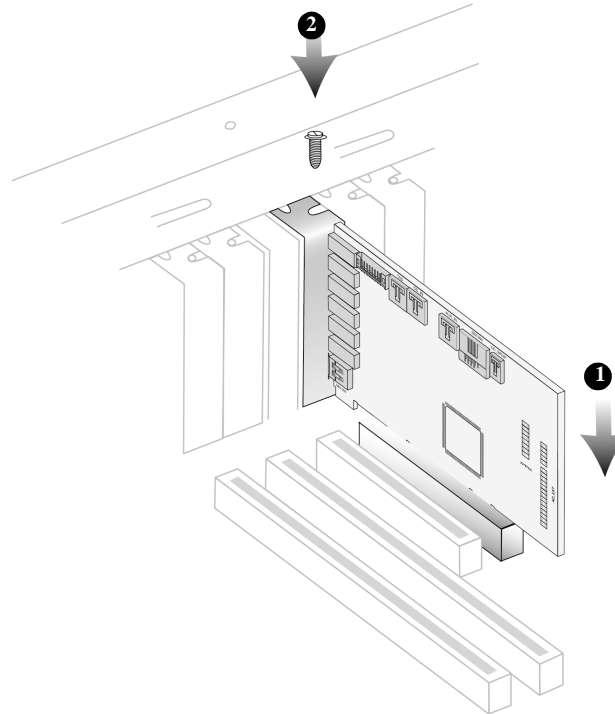
그림 1-4: 확장 슬롯에 오디오 카드 고정하기
