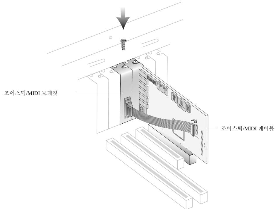
그림 1-5: 확장 슬롯에 오디오 카드 고정하기
