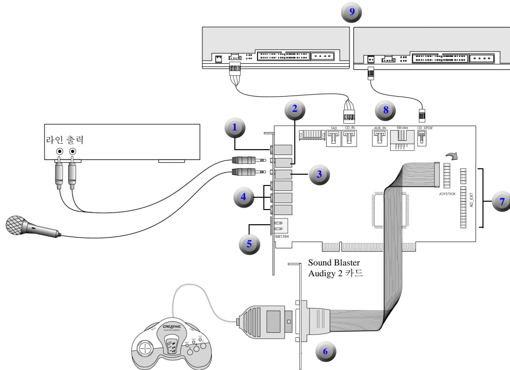
그림 1-7: 기타 장치 연결하기
